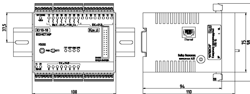
Рисунок 1.3. Габаритные и установочные размеры базового блока K110
