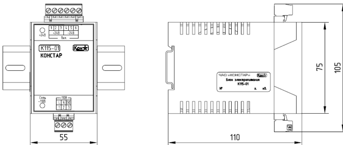
Рисунок 1.5. Габаритные и установочные размеры блока питания K115
