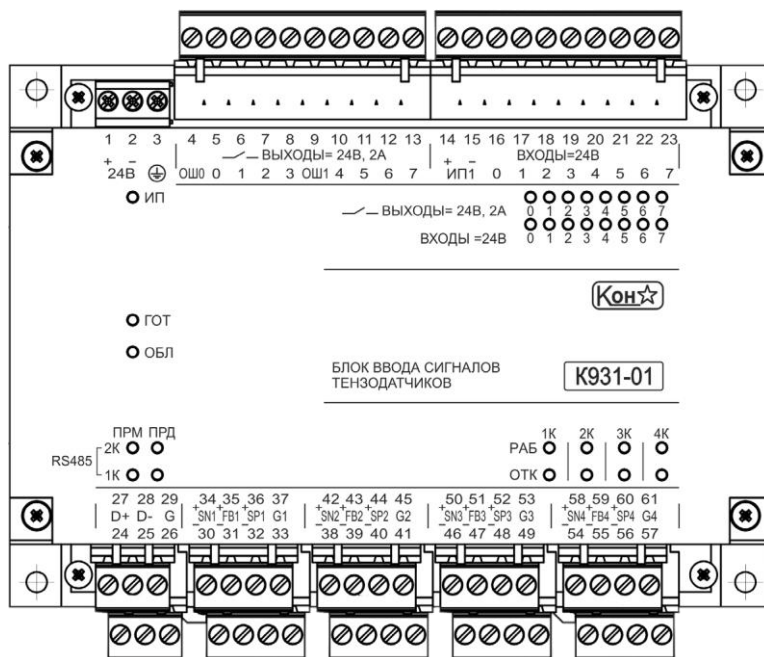
На рисунке 1 приведена лицевая панель блока ввода сигналов тензодатчиков K931-01 .
